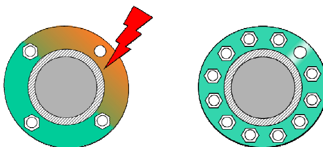
Abb.1: erhöhtes Gefahrenpotential bei Verbindungen mit 4 Schrauben
