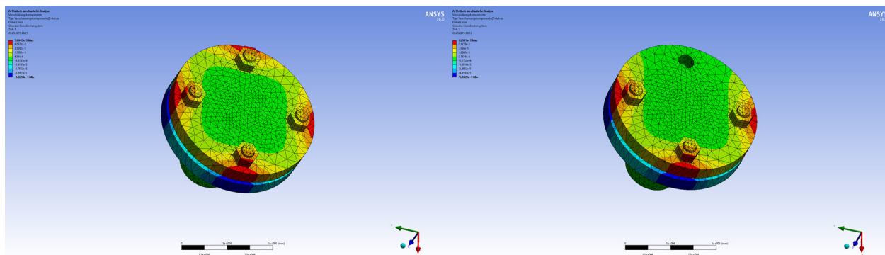
Abb.2: Abbildung der Spannungen an einer Flanschverbindung nach DIN EN 1092-1, Vorschweißflansch(Typ 11) mit Blinddeckel(Typ 05) DN50 PN40, Druck 40bar links mit 4 Schrauben und rechts mit einer fehlenden Schraube
