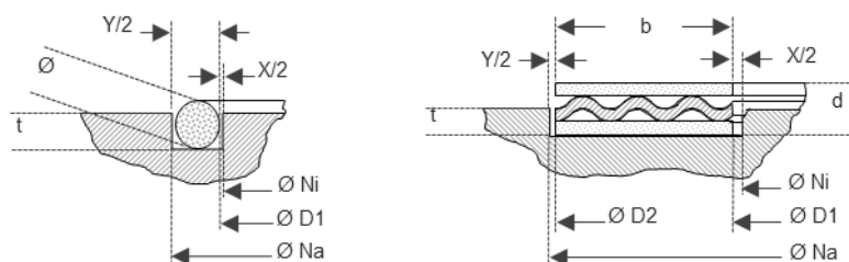
Abb.6: Vermassung der Nuten und Dichtungen links O-Ring, rechts Flachdichtung
