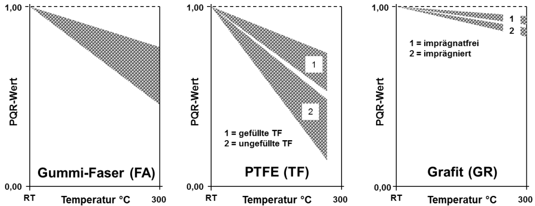
Abb.1: Schraubenkraftverlust dargestellt anhand der P_{QR} -Werte nach EN 13555
