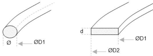
Abb.5: Vermassung von Dichtungen
