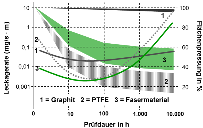
Abb.2: Darstellung des Zusammenhanges von Leckage und Schraubenkraftverlust
