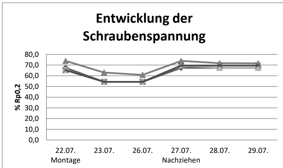
Abb.6: Darstellung der Entwicklung der Schraubenauslastung
