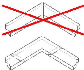
Abb.4: Ausführung der Ecke
